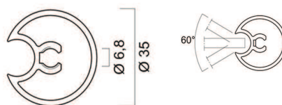
Profil rainuré diam. 35 07.052.1202.11 / 12 dim. 5000 x 35mm
