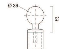
Embout boule à visser 07.414.5518.11 / 12
