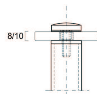
Embout pour glace percée 07.414.5570.11 / 12
