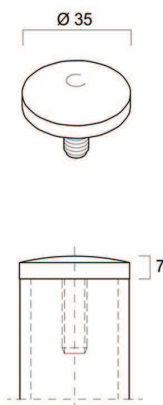
Embout à visser 07.414.5519.11 / 12
